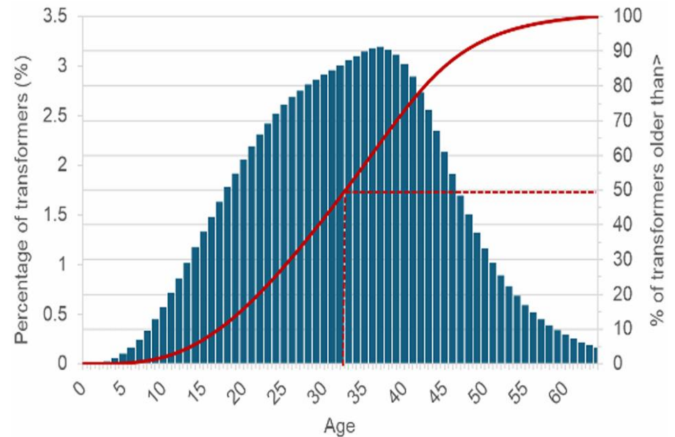
미국 내 중저압·배전용 변압기 연령(2023년 기준)
